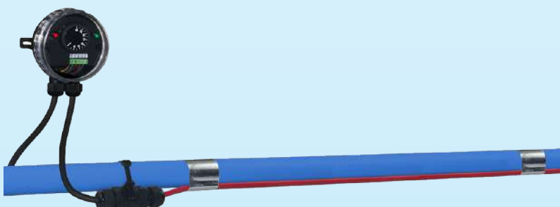
Exemple de montage en commande d'un câble chauffant pour mise hors gel d'un tuyau en PVC, combiné avec un boîtier Y24.
