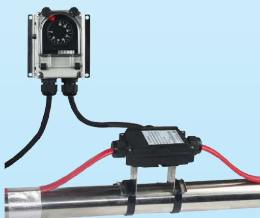
Exemple de montage en commande de deux câbles chauffants pour mise hors gel d'un tuyau, combiné avec un boîtier Y26 avec platine de surélévation
